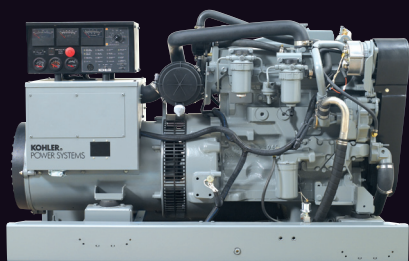
40EOZC 40 kW
