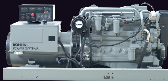
99EOZC 99 kW
